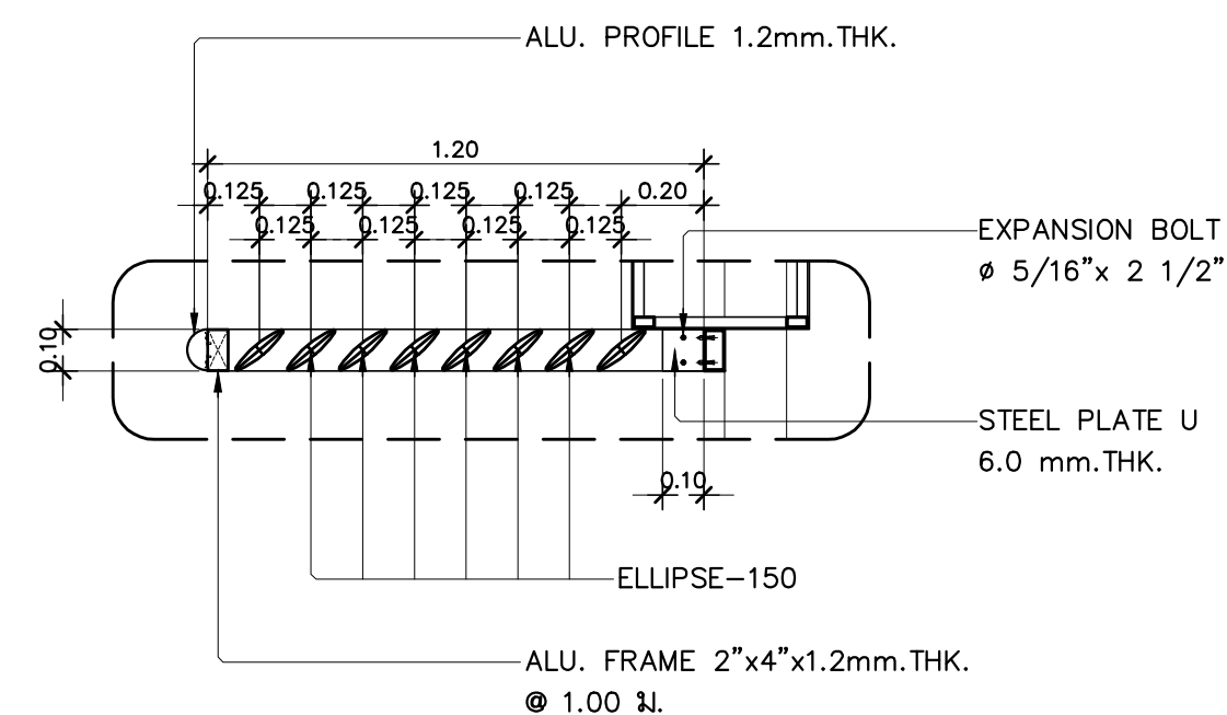
แบบขยายรูปตัด DT7 มาตราส่วน 1:20
