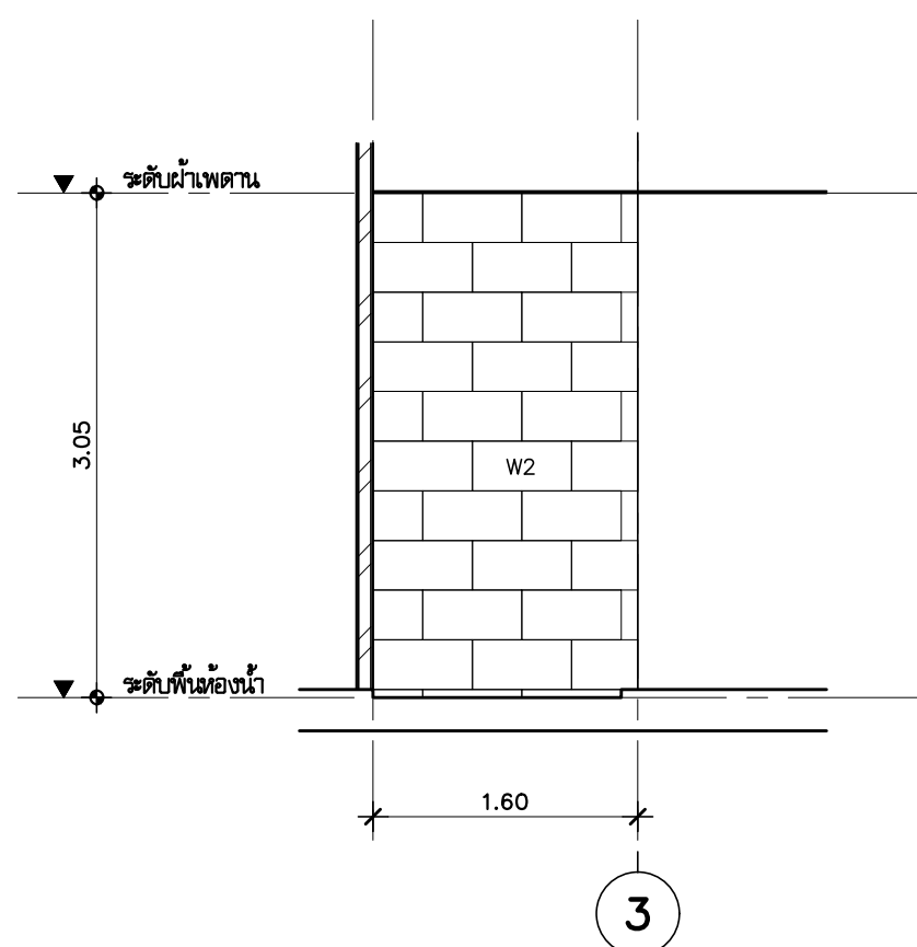
แบบขยาย SH1 ( รูปตัด A ) มาตราส่วน 1:50
