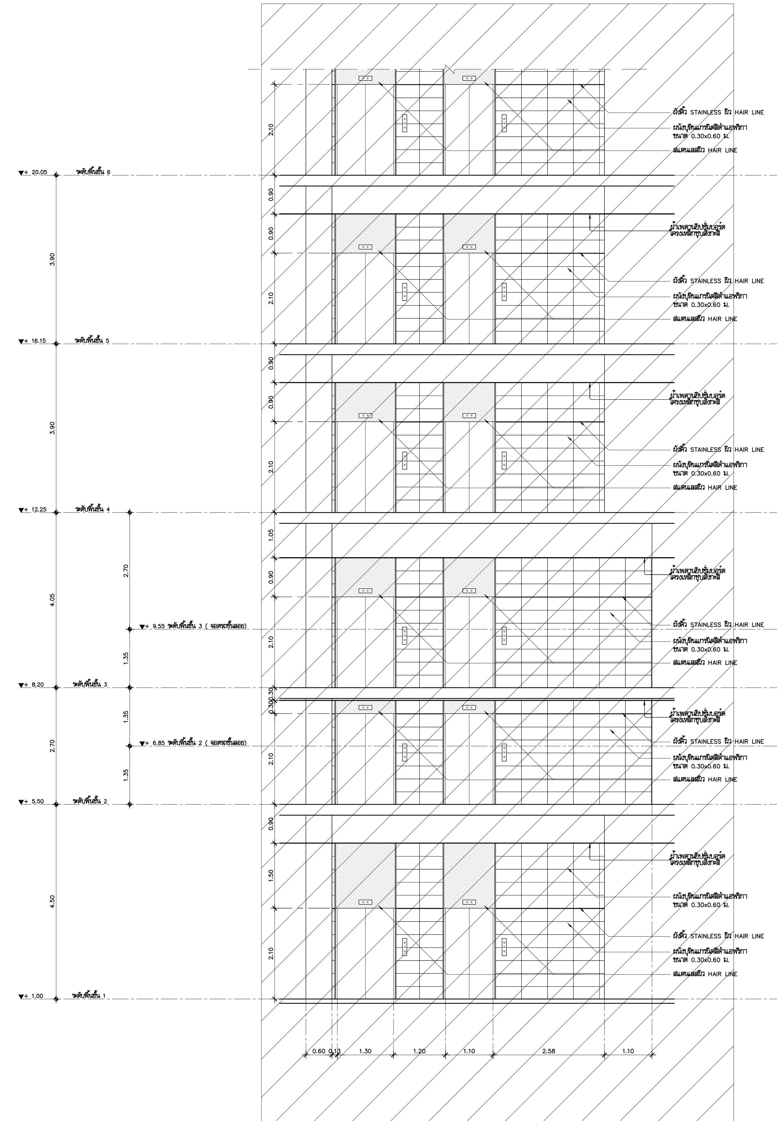
แบบขยายรูปด้านลิฟต์ L1 (ส่วนที่1) มาตราส่วน 1:50
