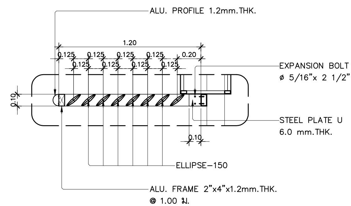
แบบขยายรูปตัด DT7 มาตรฐาน 1:20
