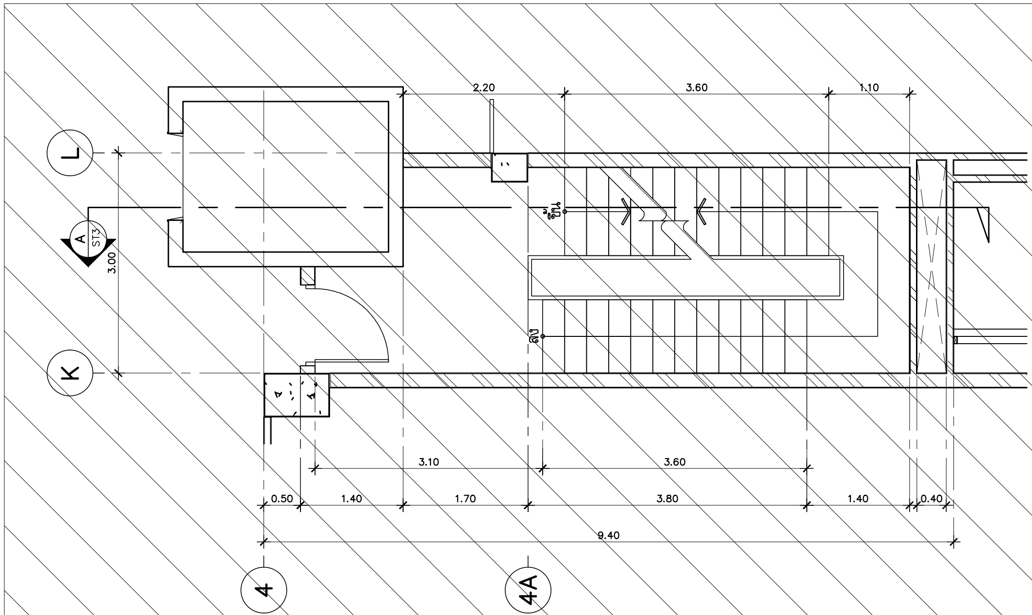
แปลนขยายบันได ST3 ชั้น 8-10
