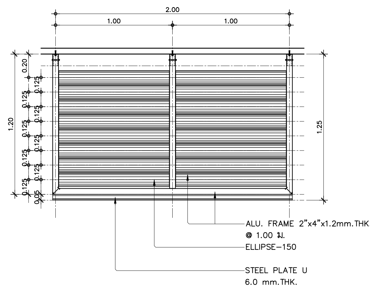
แบบขยาย DT6 มาตราส่วน 1:20
