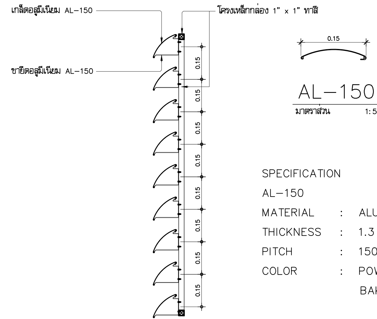
SECTION มาตราส่วน 1:10
