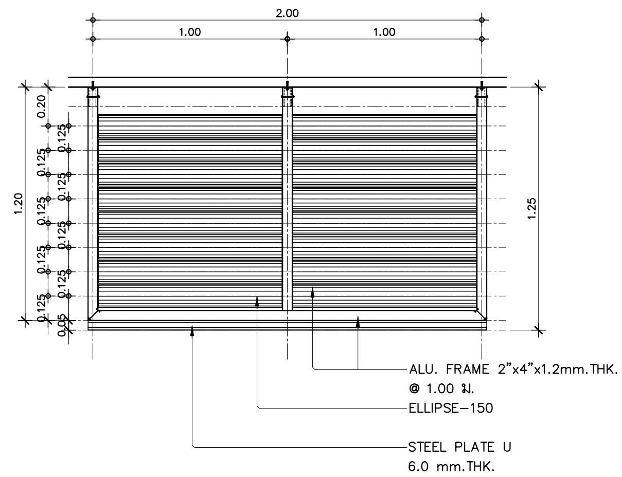
แบบขยาย DT7 มาตรฐาน 1:20
