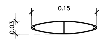
แบบขยาย ELLIPSE-150 มาตรฐาน 1:5
