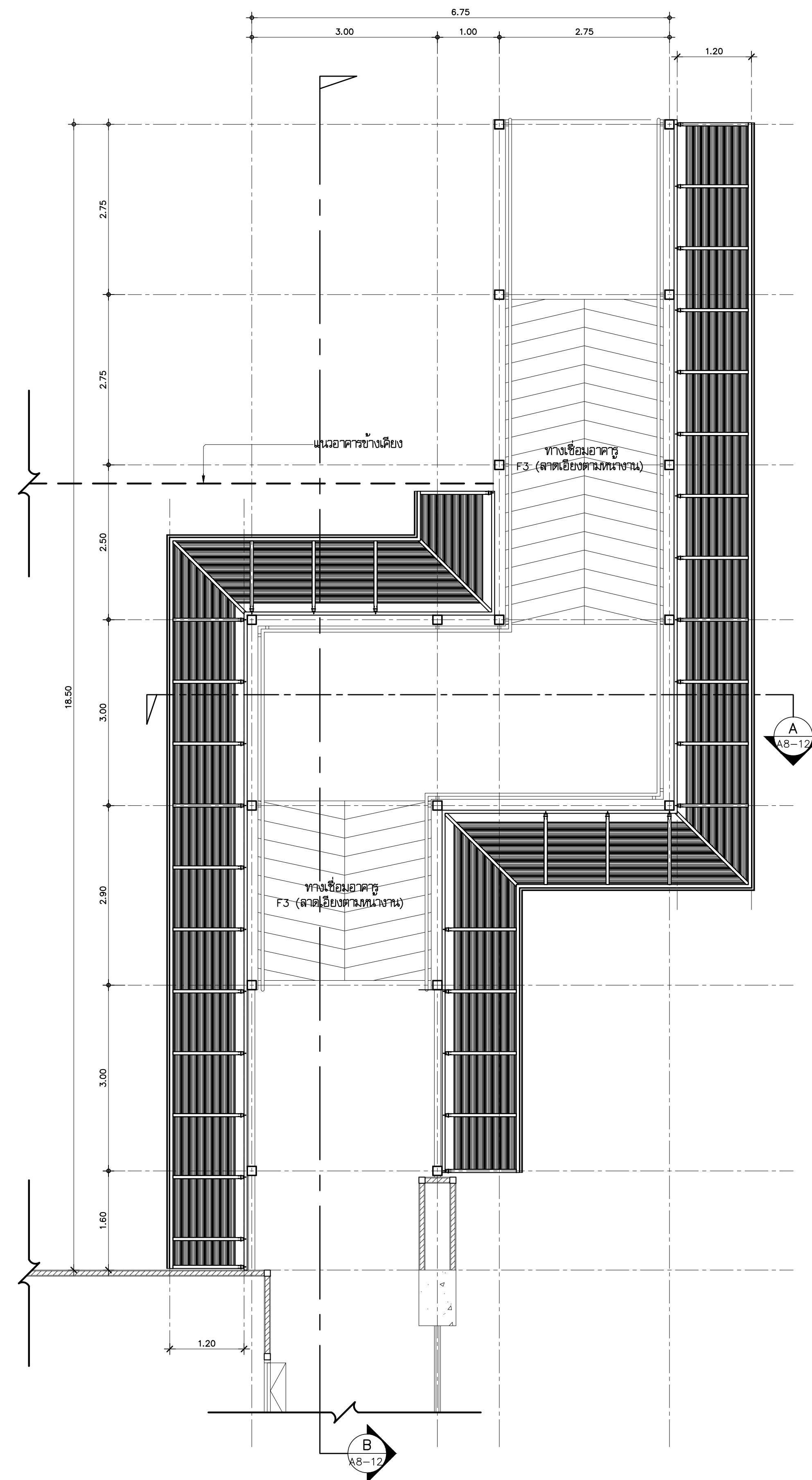
แบบขยายแปลน BR2 พื้นชั้น 4 มาตราส่วน 1:50
