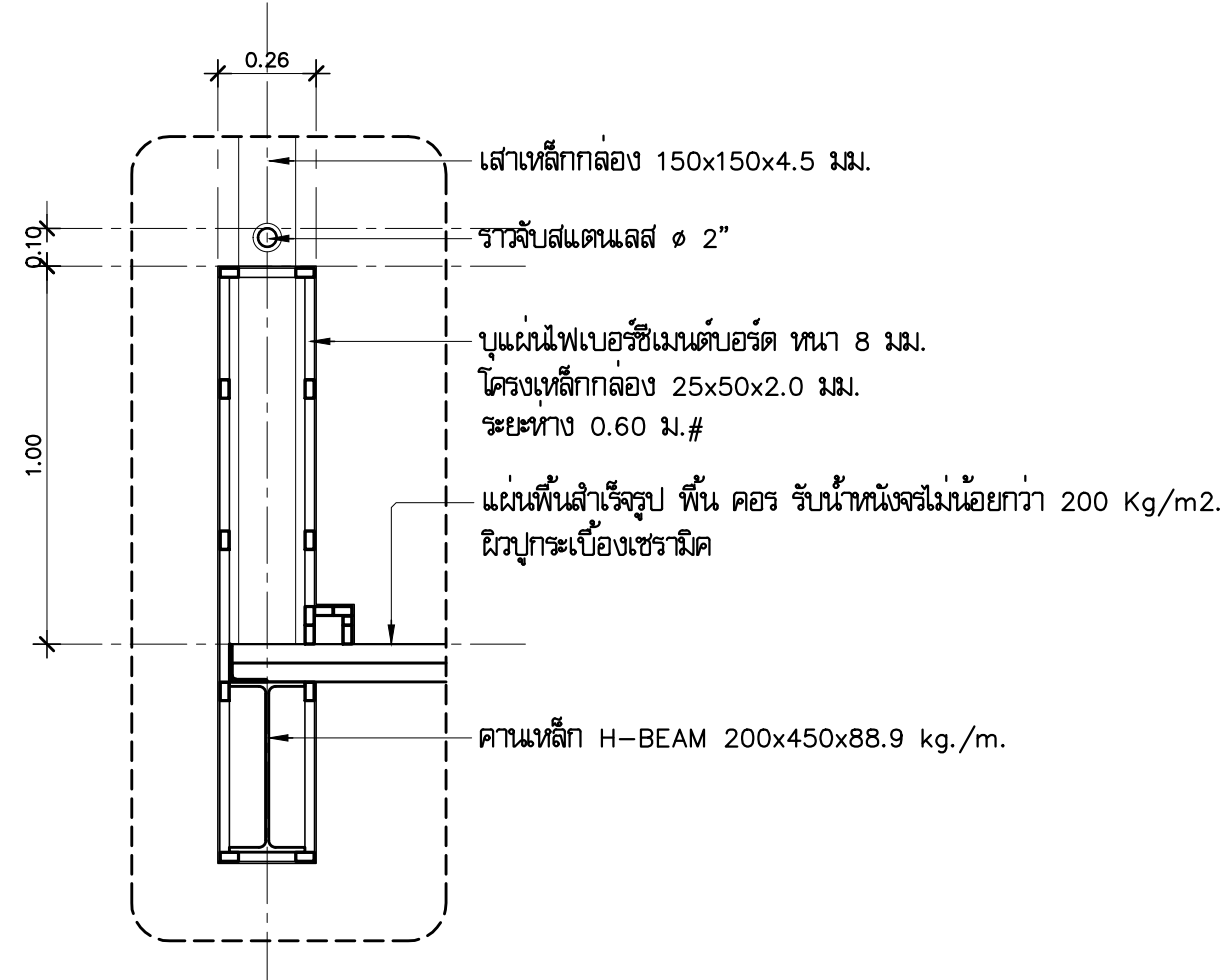
แบบขยาย DT6 มาตรฐาน 1:20
