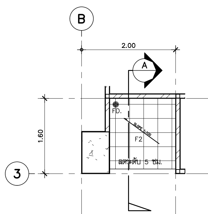
แบบขยาย SH1 ( แปลน ) มาตราส่วน 1:50
