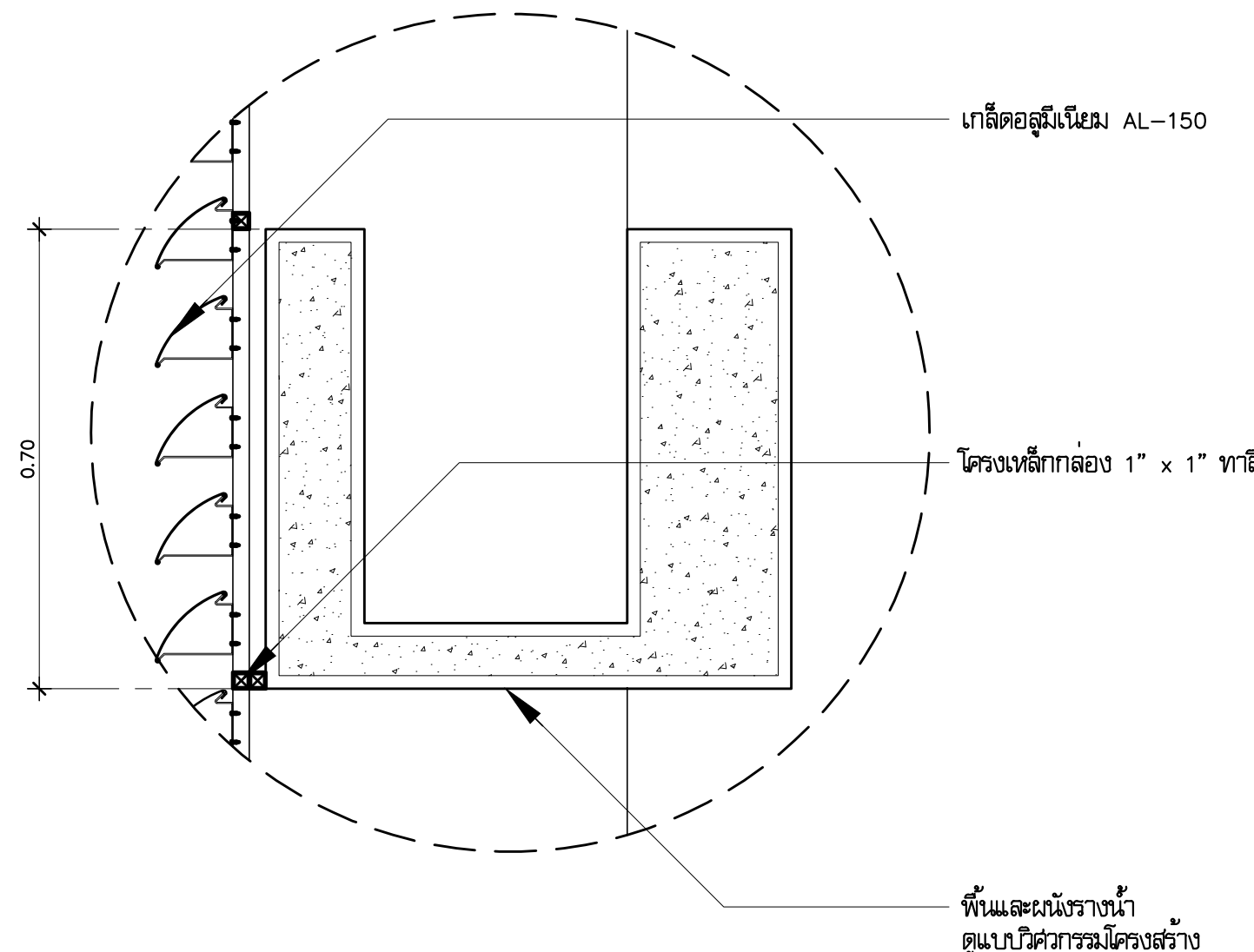
แบบขยาย DT7 มาตราส่วน 1:10
