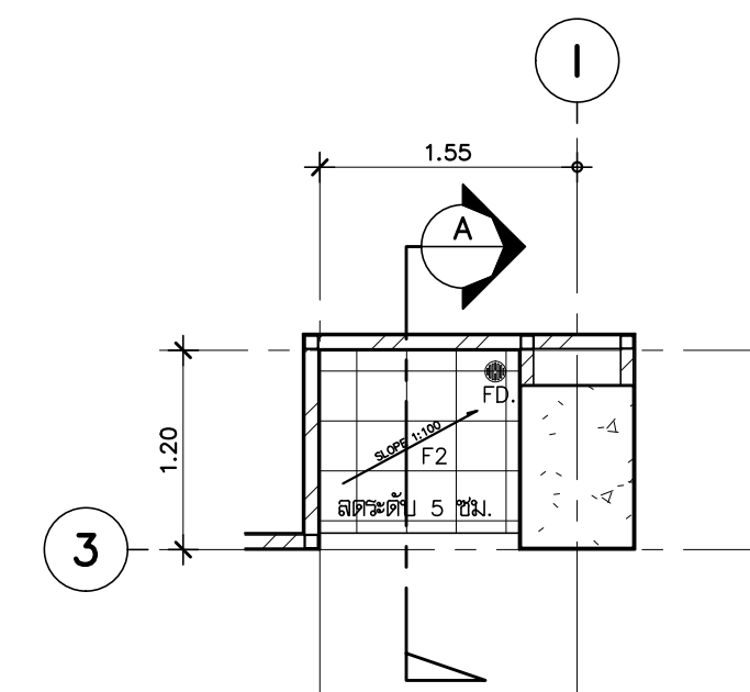
แบบขยาย SH2 ( แปลน ) มาตราส่วน 1:50
