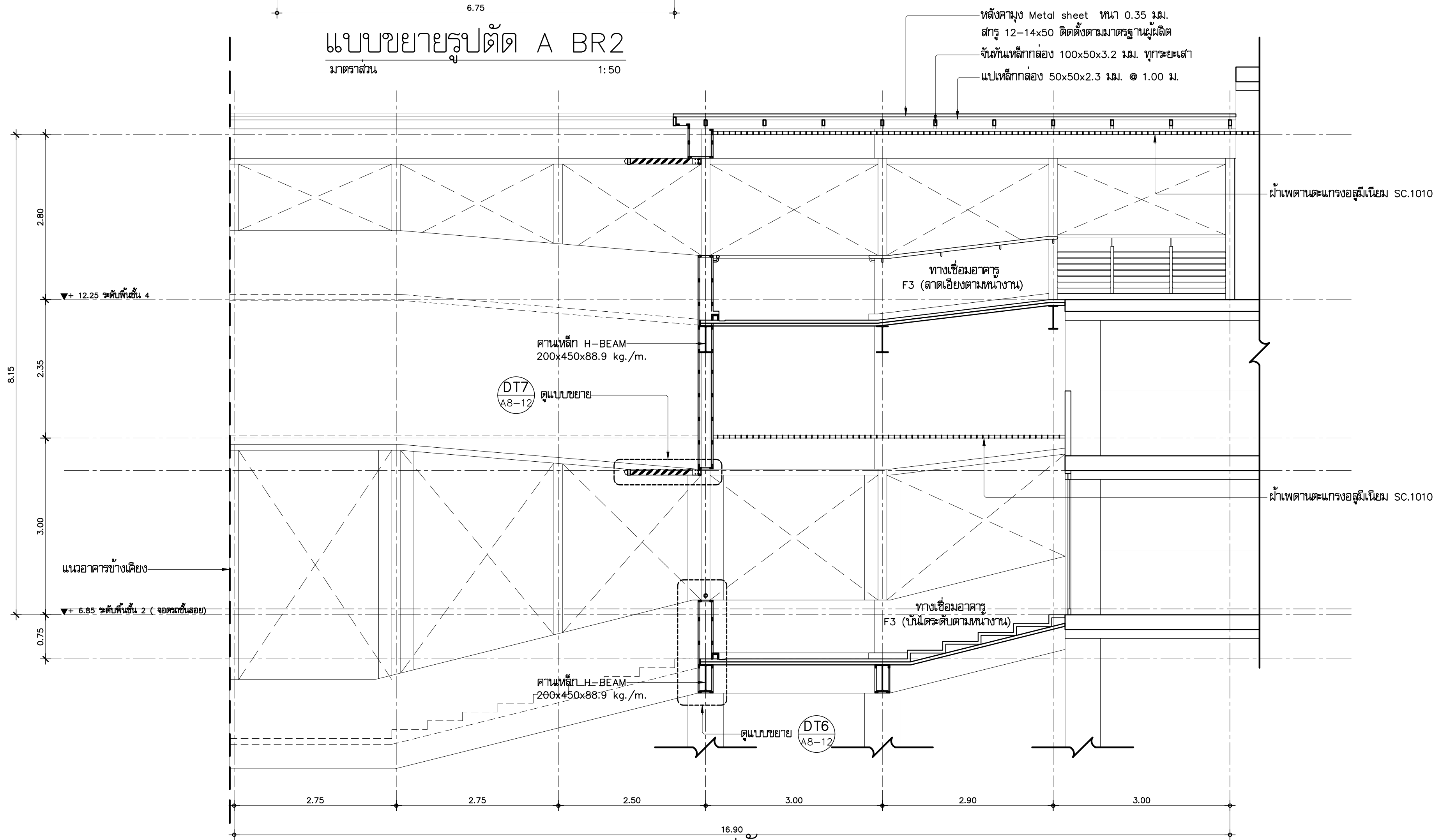
แบบขยายรูปตัด B BR2 มาตรฐาน 1:50
