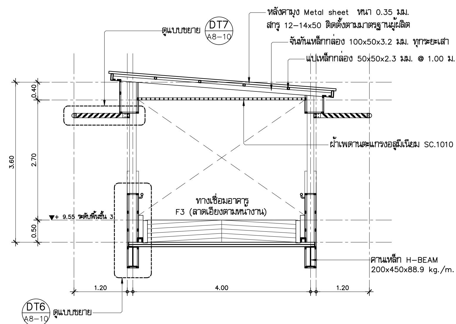
แบบขยายรูปตัด A BR1 มาตราส่วน 1:50
