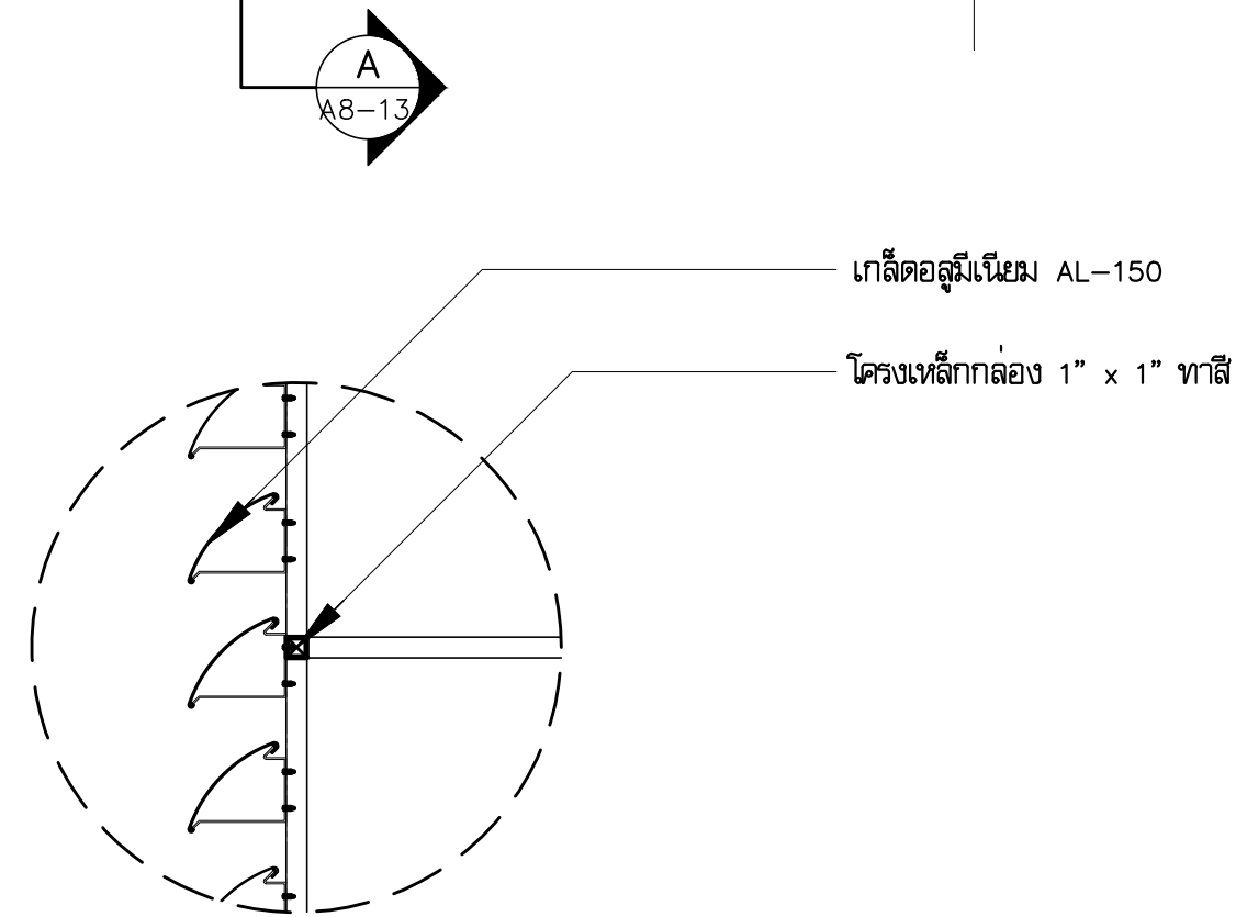
แบบขยาย DT6 มาตราส่วน 1:10
