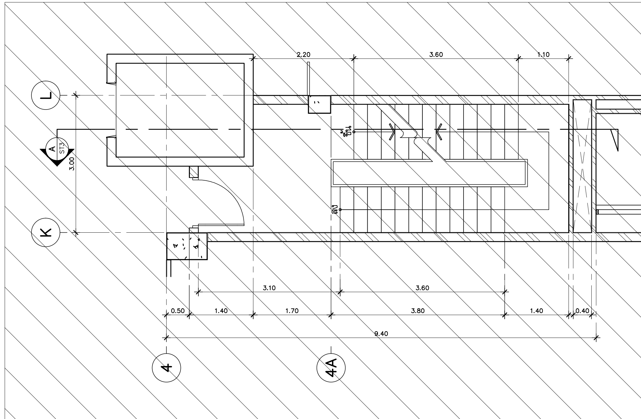
แปลนขยายบันได ST3 ชั้น 8-10
