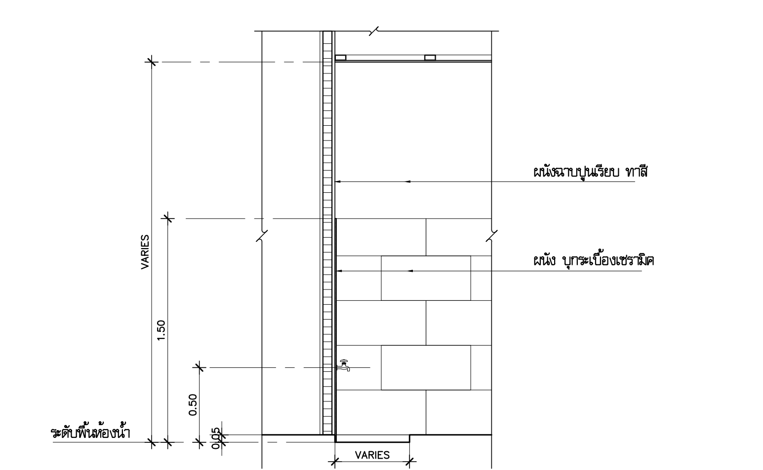
แบบขยายบ่อชักล้าง DT-4 1: 25
