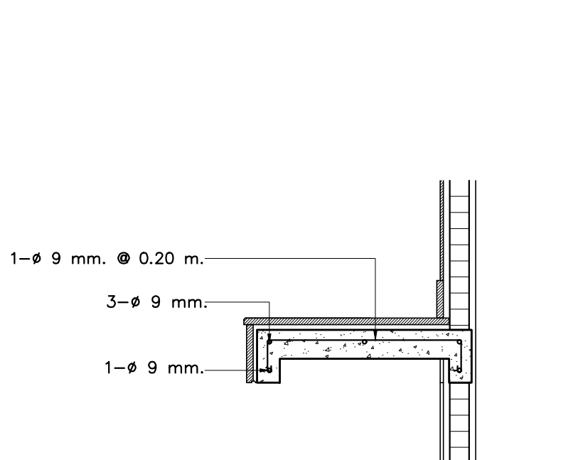
แบบขยายการเสริมเหล็กเคาน์เตอร์
