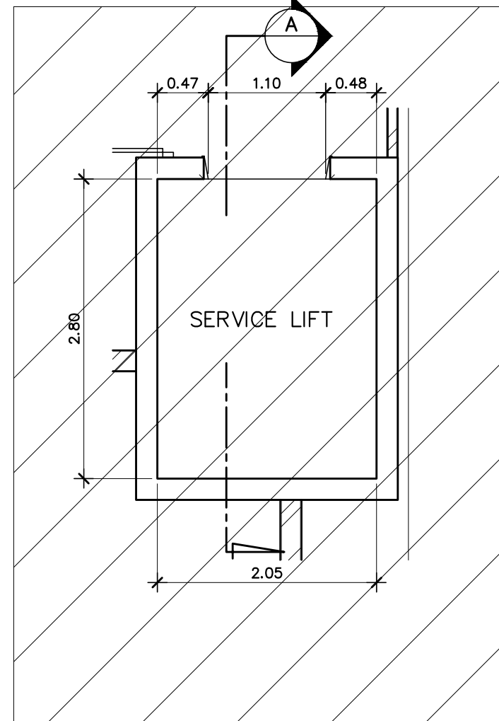
แปลนชั้น 1 ลิฟต์ LI2 มาตราส่วน 1:50
