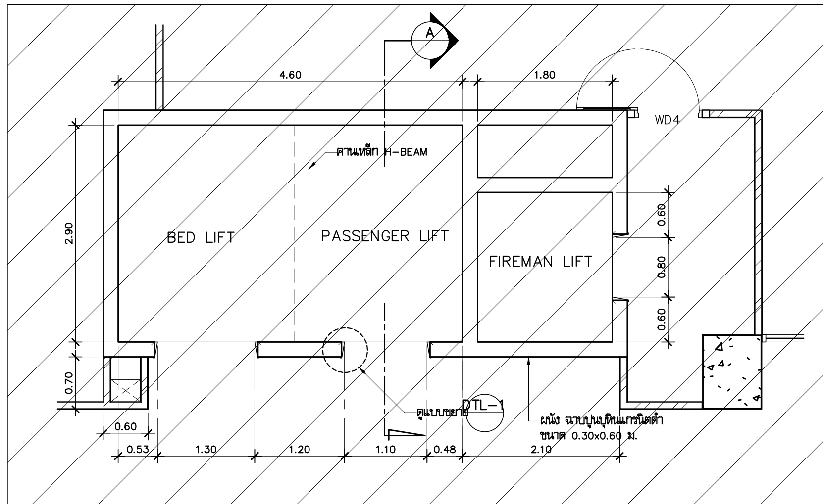
แปลนชั้น 4 ลิฟต์ LI1 มาตราส่วน 1:50
