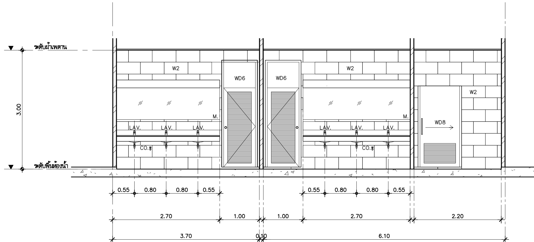
แบบขยาย WC4 ( รูปตัด A ) มาตราส่วน 1:50
