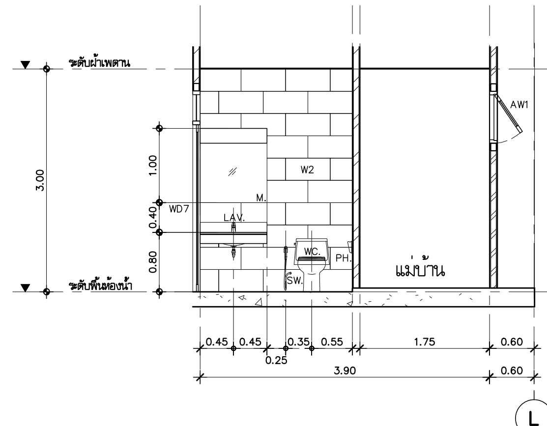
แบบขยาย WC7 ( รูปตัด D ) มาตราส่วน 1:50
