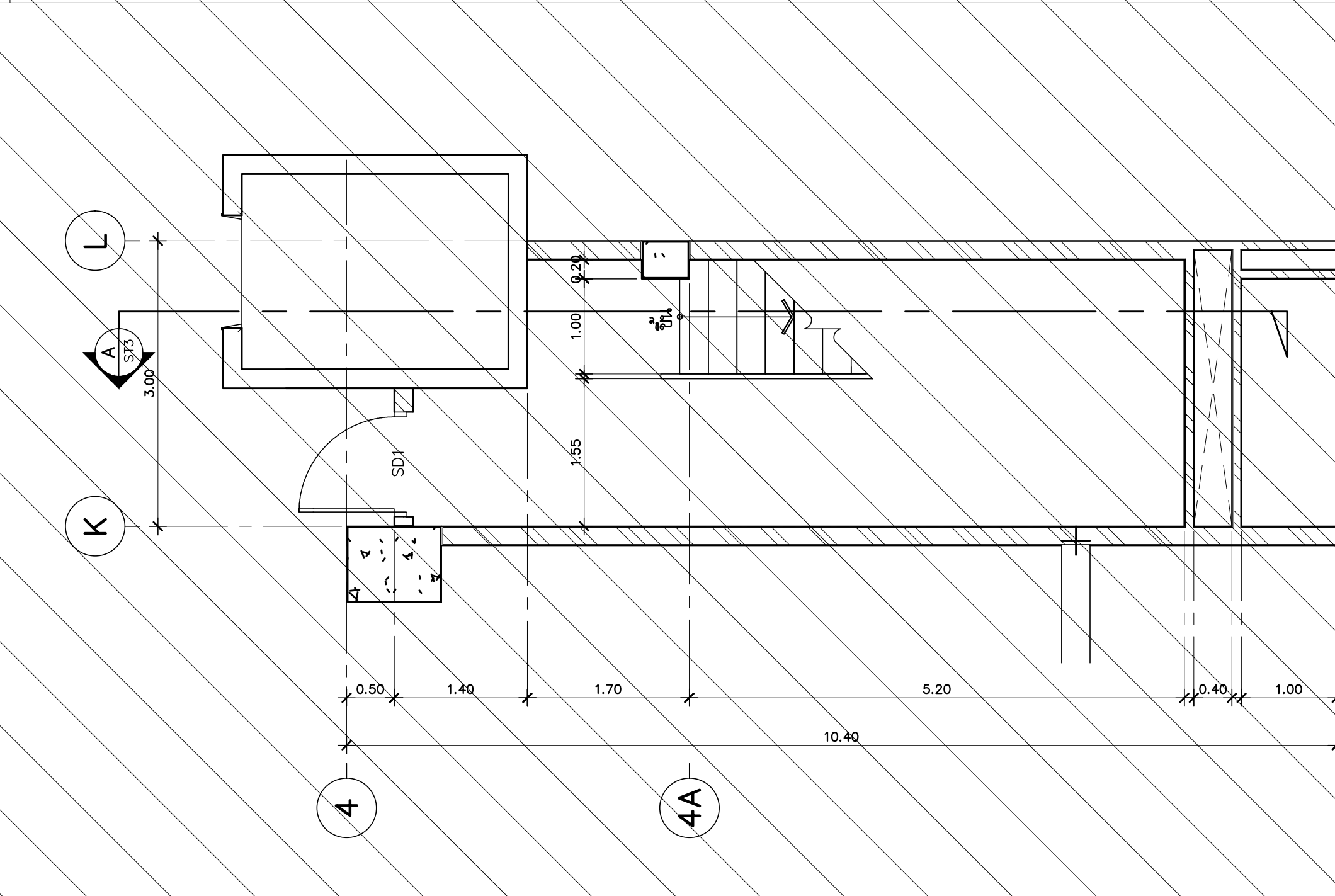
แปลนขยายบันได ST3 ชั้น 8-10
