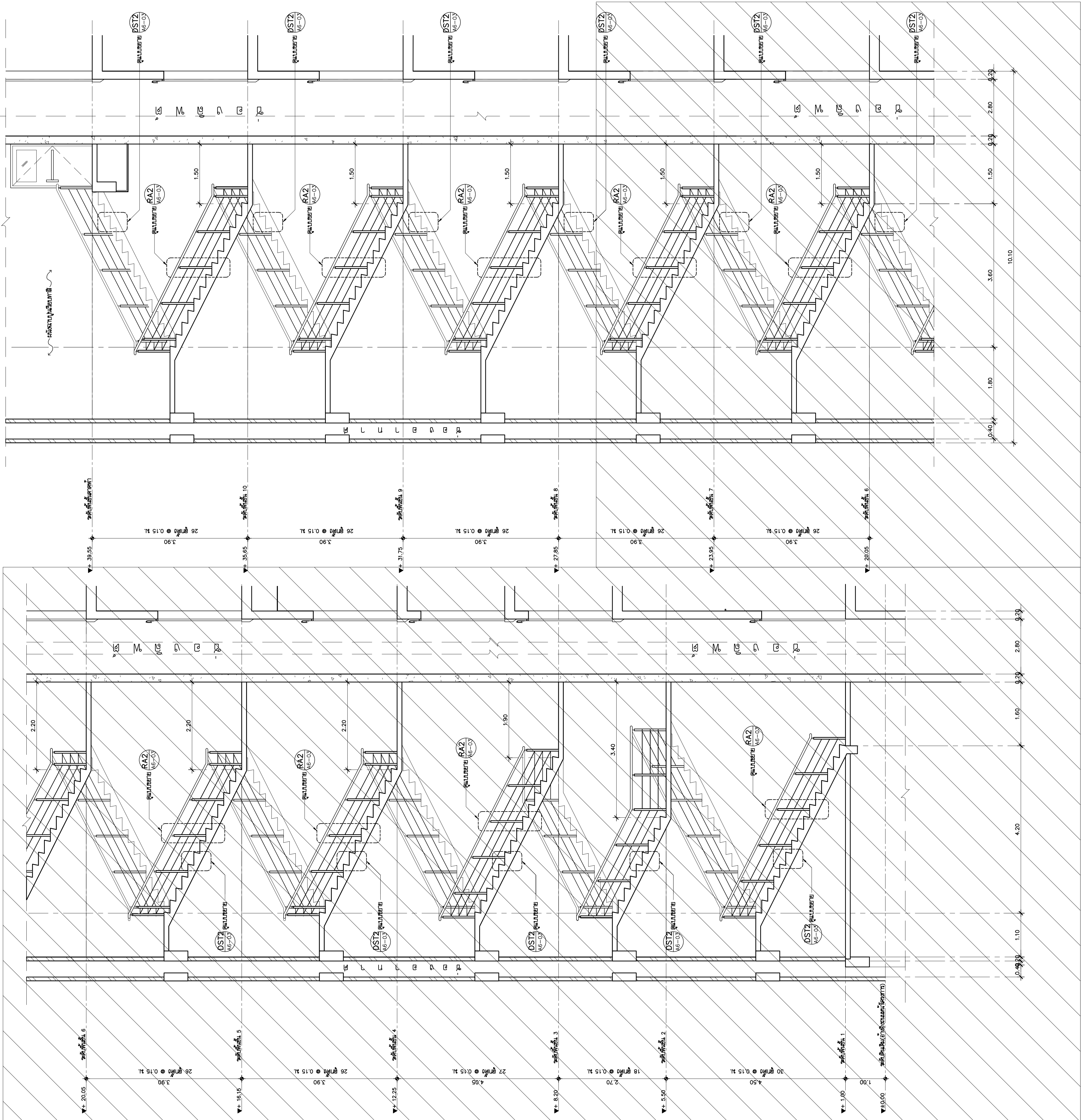
แบบขยายบันได ST3 รูปตัด A (ส่วนที่2) มาตราส่วน 1:50
