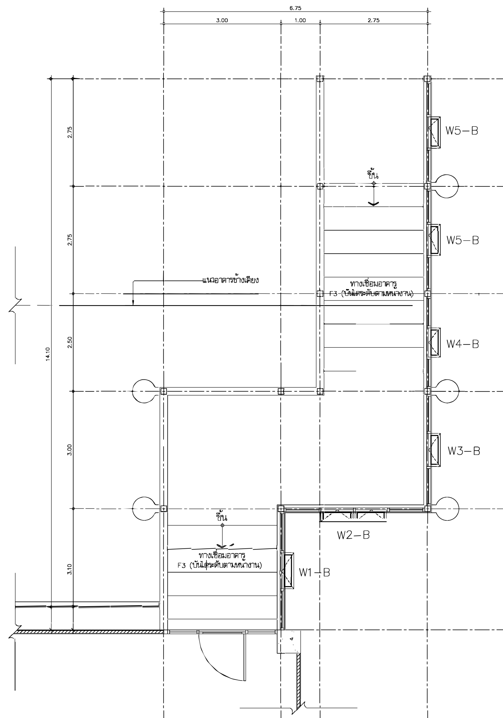
แบบขยายแปลน BR2 พื้นชั้น 2 มาตราส่วน 1:50
