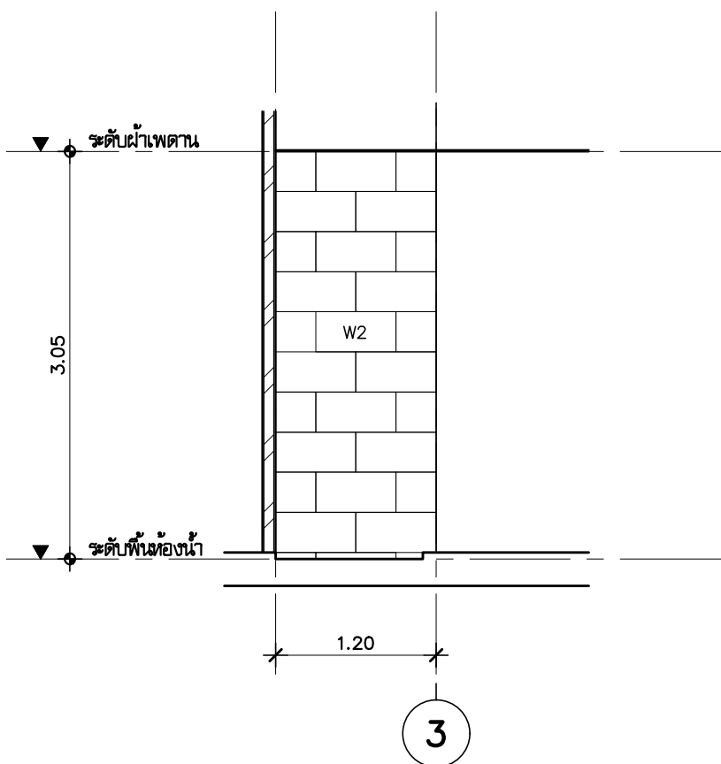
แบบขยาย SH2 ( รูปตัด A ) มาตราส่วน 1:50
