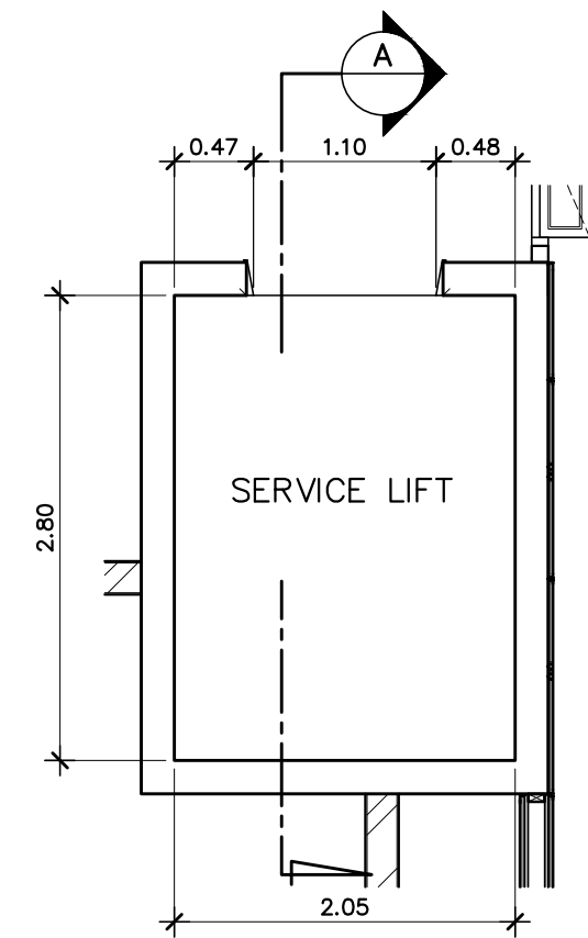
แปลนชั้น 2-3 ลิฟต์ LI1 มาตราส่วน 1:50
