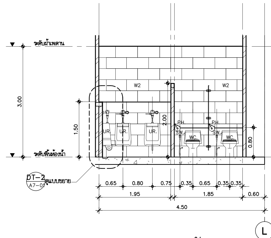
แบบขยาย WC7 ( รูปตัด B ) มาตราส่วน 1:50
