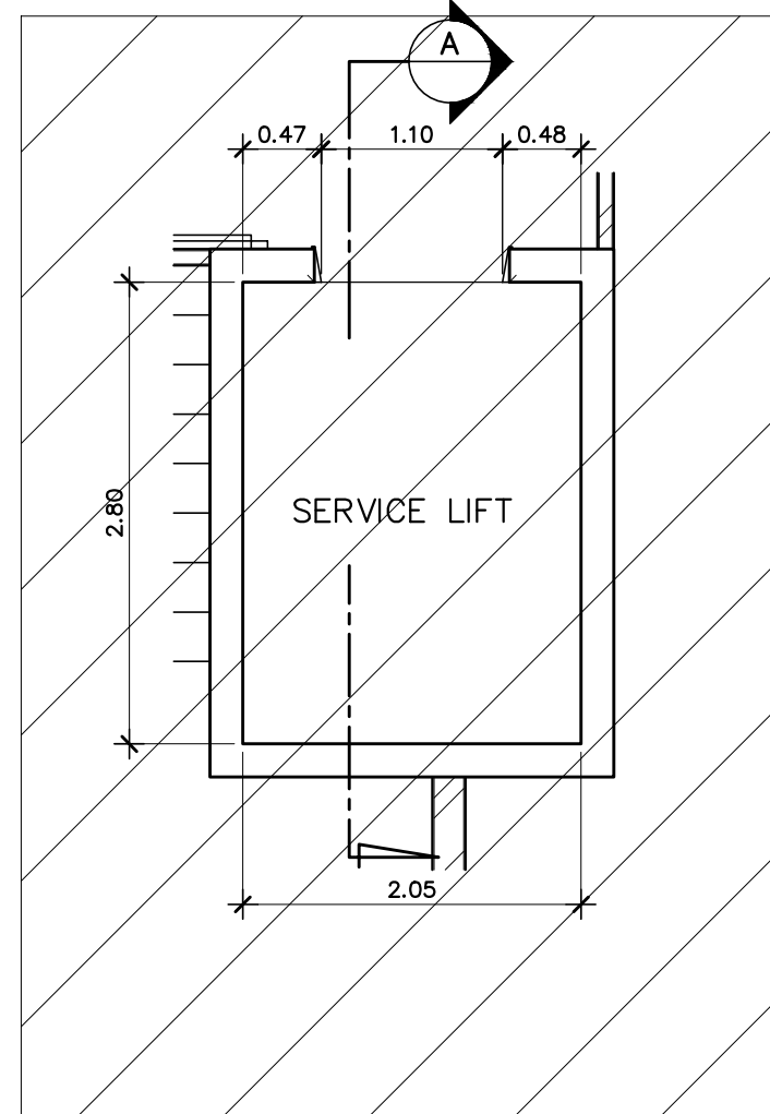
แปลนชั้น 2-3 ลิฟต์ LI1 มาตราส่วน 1:50
