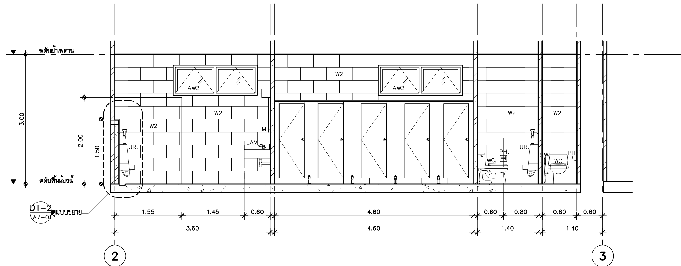
แบบขยาย WC7 ( รูปตัด A ) มาตราส่วน 1:50
