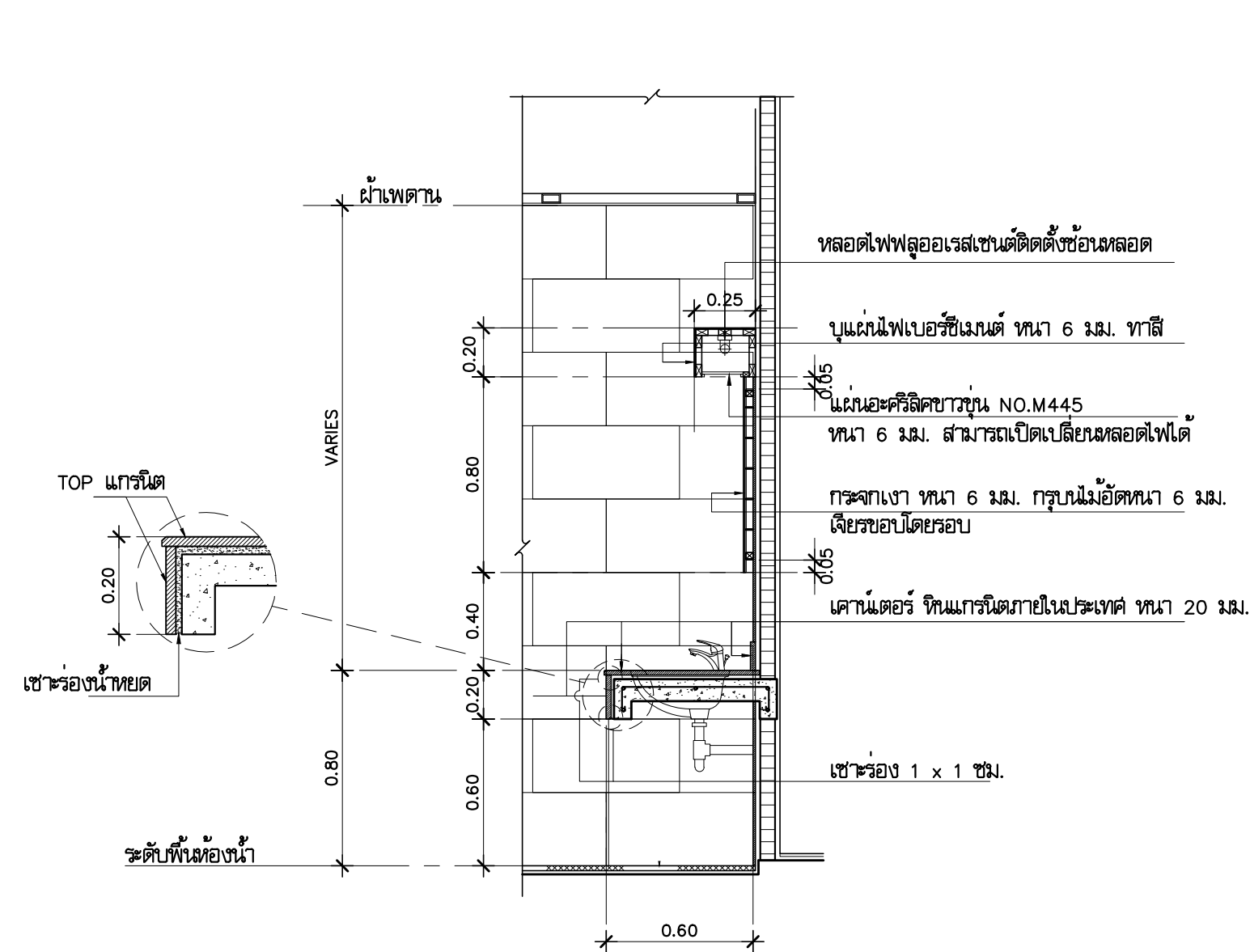
แบบขยายเคาน์เตอร์ DT-1 1: 25
