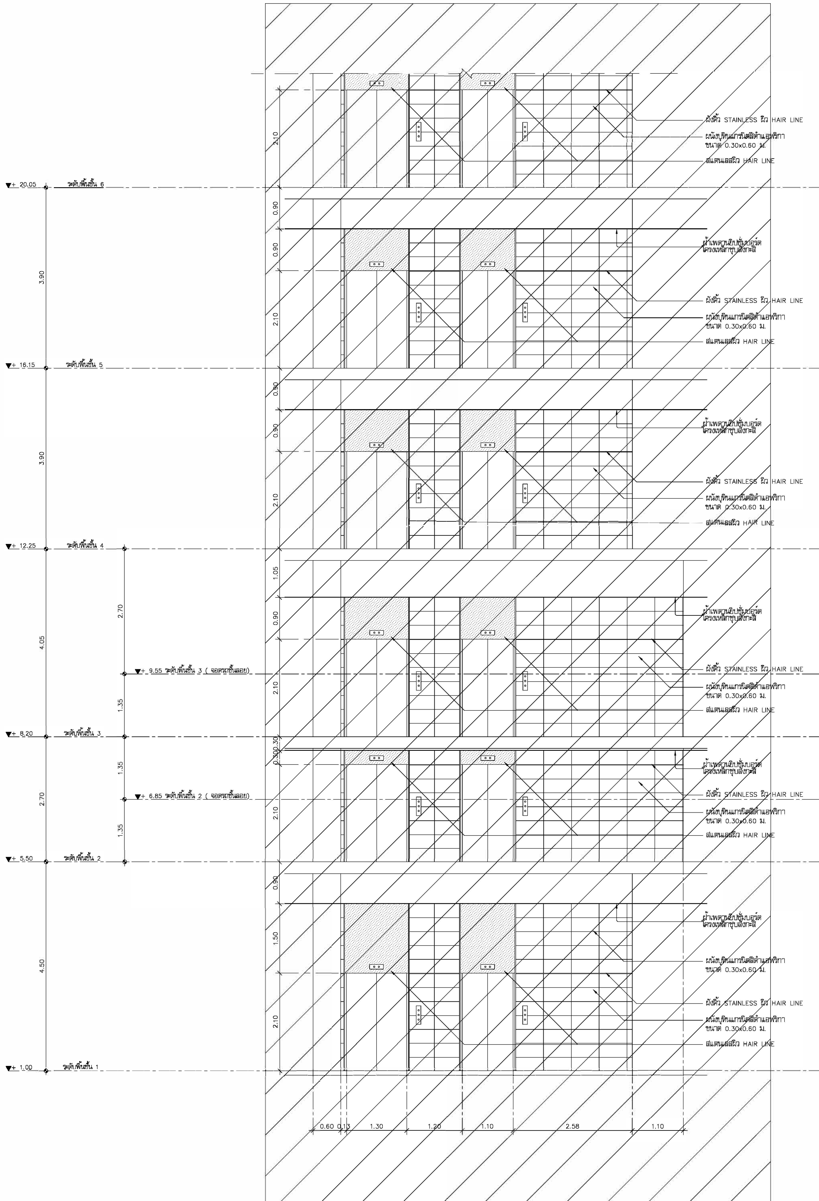
แบบขยายรูปด้านลิฟต์ L1 (ส่วนที่1) มาตราส่วน 1:50
