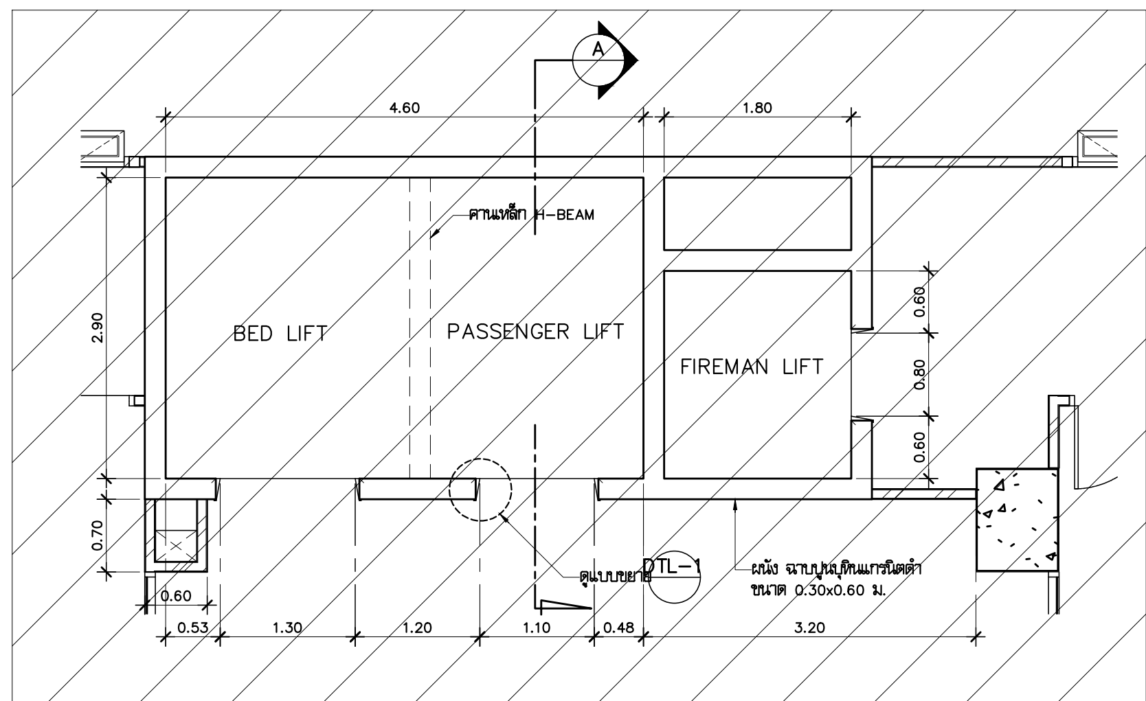
แปลนชั้น 2-3 ลิฟต์ LI1 มาตราส่วน 1:50
