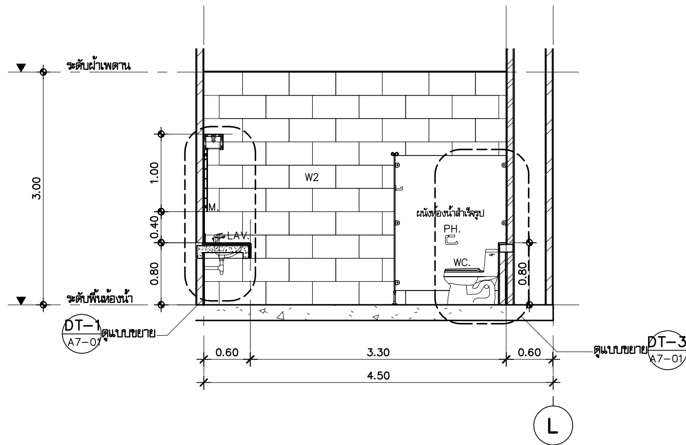
แบบขยาย WC7 ( รูปตัด C ) มาตราส่วน 1:50
