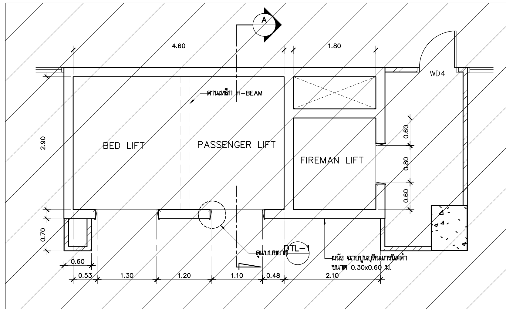
แปลนชั้น 1 ลิฟต์ LI1 มาตราส่วน 1:50
