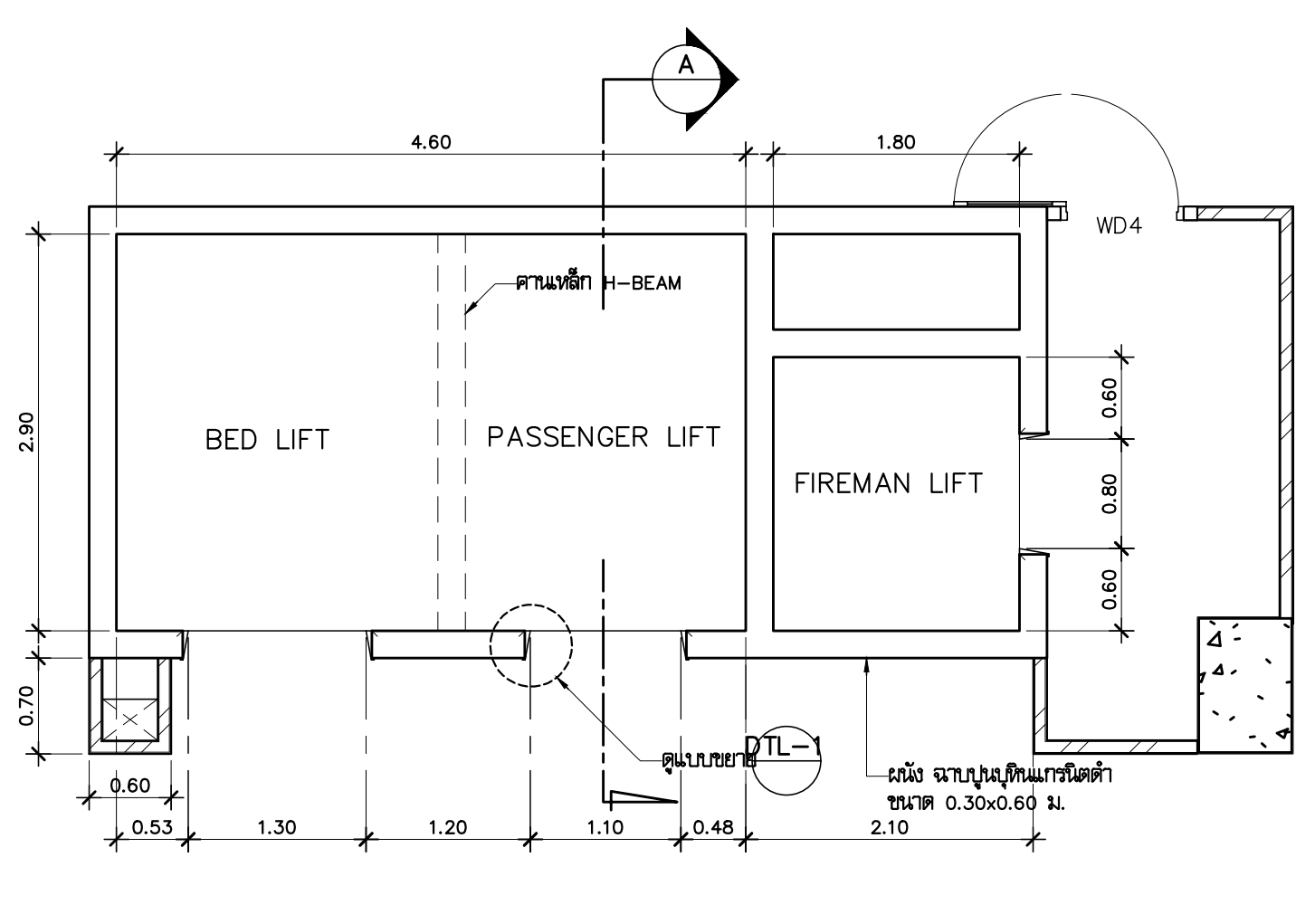
แปลนชั้น 5-10 ลิฟต์ LI1 มาตราส่วน 1:50
