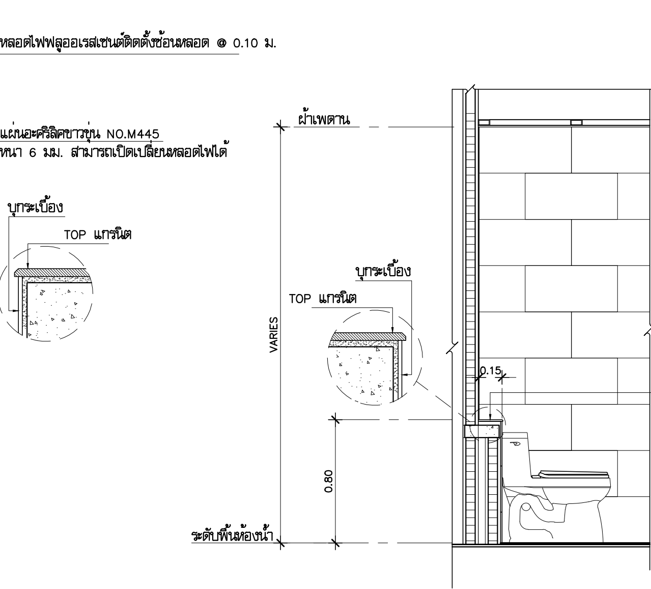
แบบขยายตำแหน่งโถส้วม DT-3 1: 25
