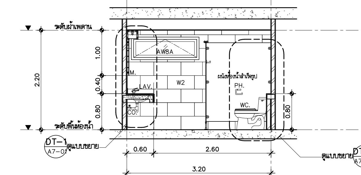
แบบขยาย WC5 ( รูปตัด B ) มาตราส่วน 1:50
