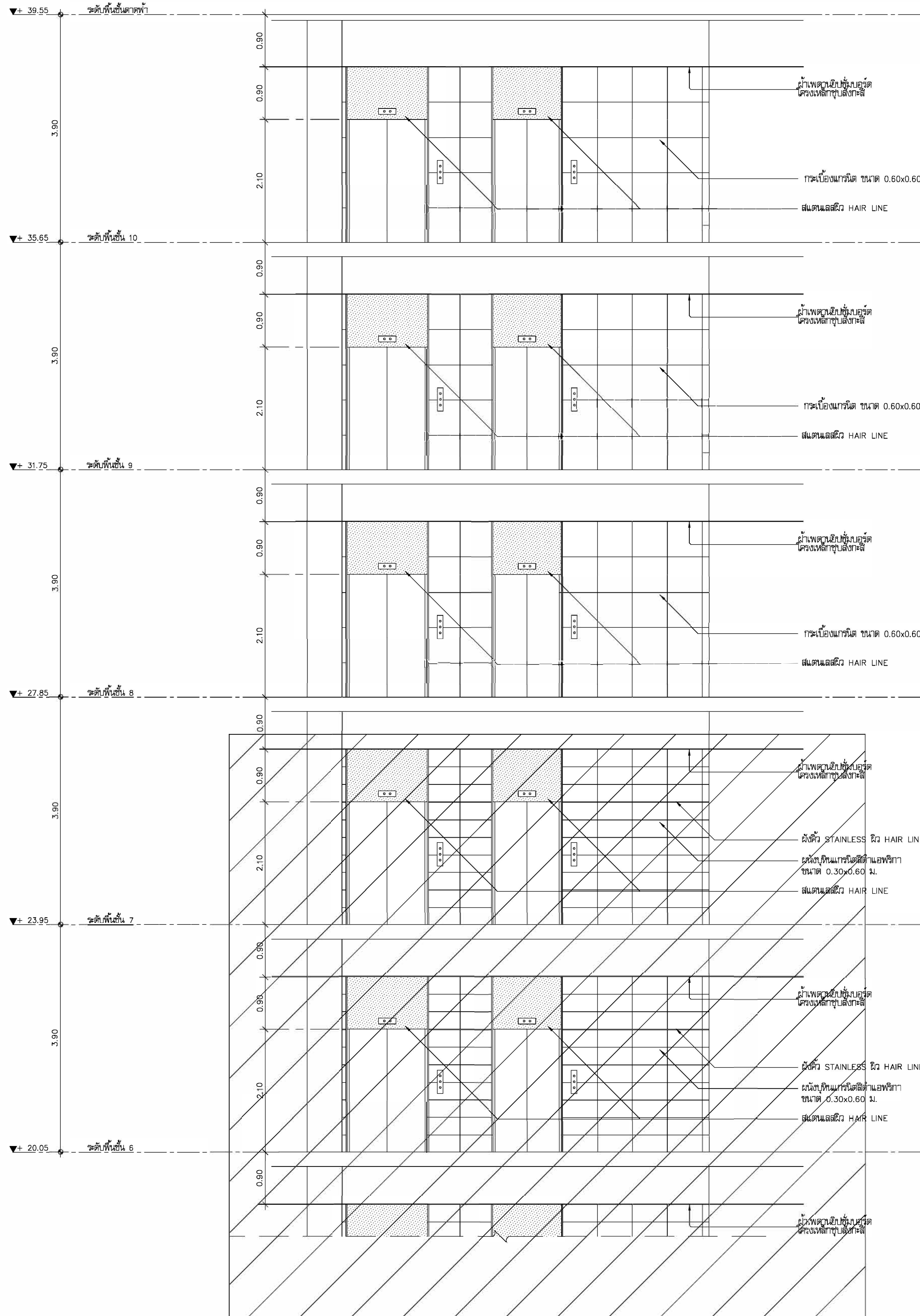
แบบขยายรูปด้านลิฟต์ L1 (ส่วนที่2) มาตราส่วน 1:50
