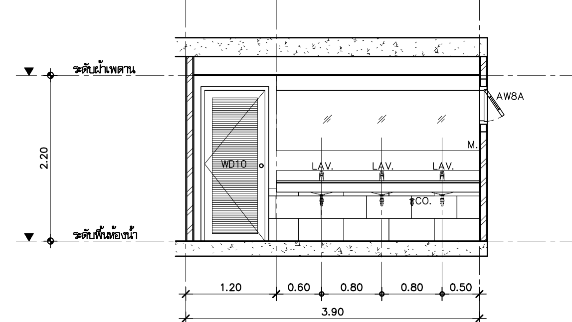
แบบขยาย WC5 ( รูปตัด A ) มาตราส่วน 1:50
