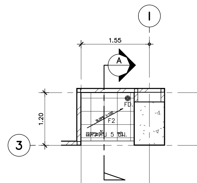
แบบขยาย SH2 ( แปลน ) มาตราส่วน 1:50
