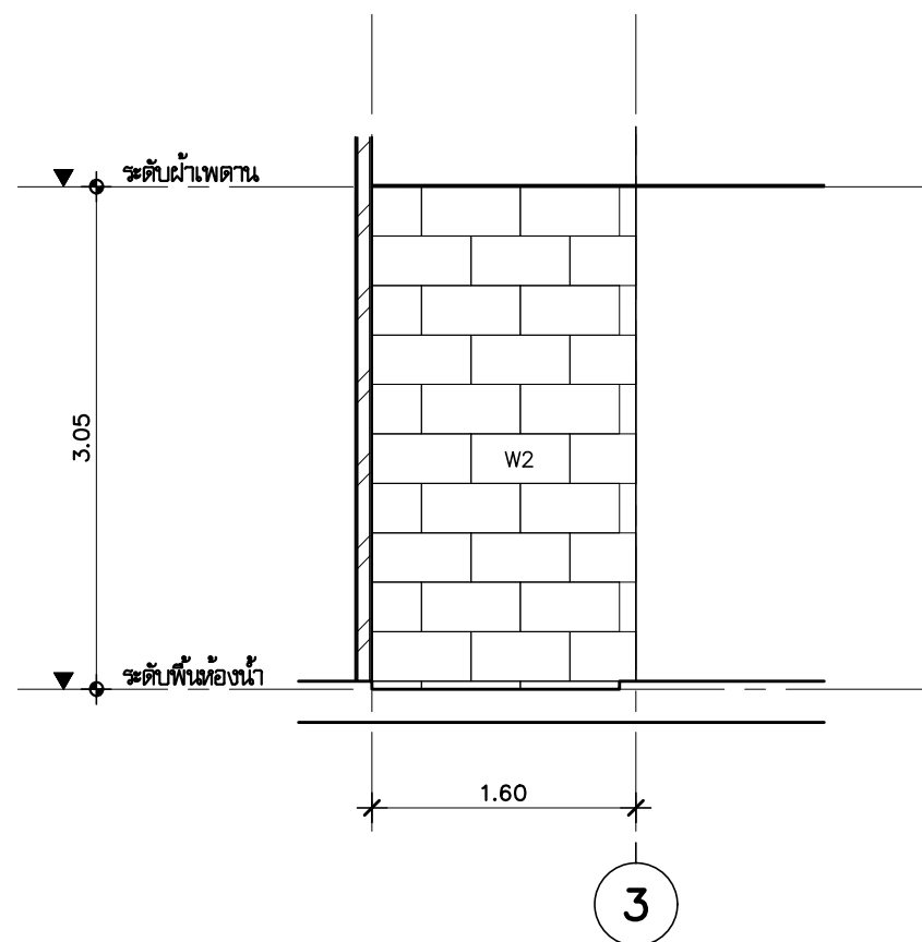
แบบขยาย SH1 ( รูปตัด A ) มาตราส่วน 1:50
