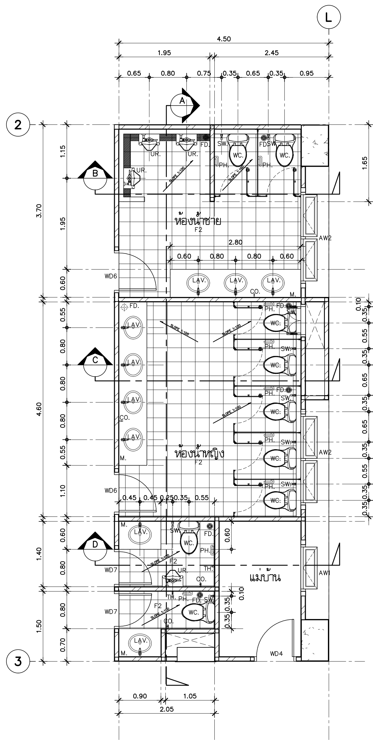
แบบขยาย WC7 ( แปลน ) มาตราส่วน 1:50
