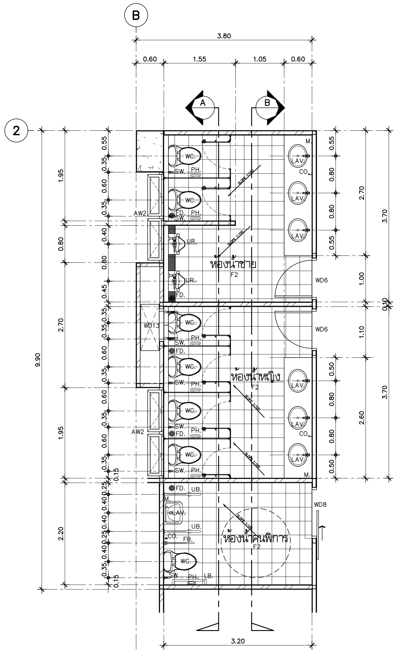
แบบขยาย WC4 ( แปลน ) มาตราส่วน 1:50
