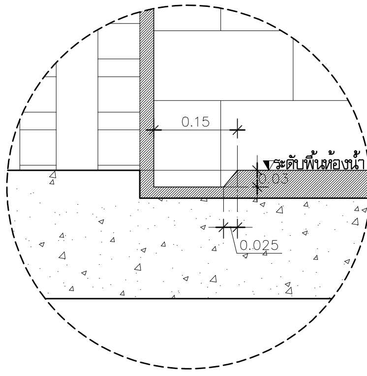
แบบขยายรางน้ำใต้โถปัสสาวะชาย มาตราส่วน 1:50
