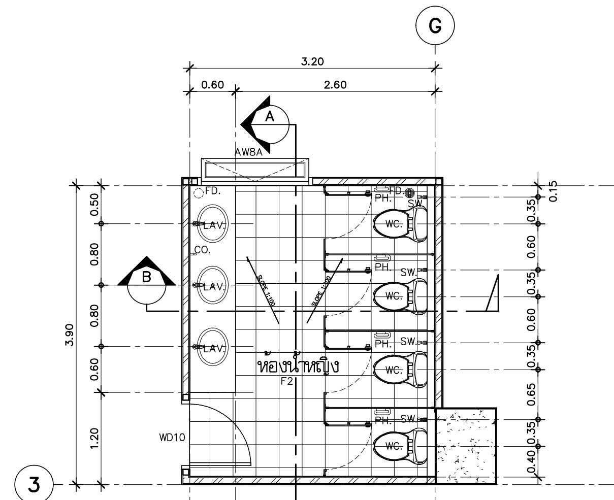
แบบขยาย WC5 ( แปลน ) มาตราส่วน 1:50
