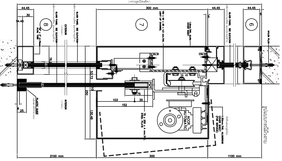
VERTICAL SECTION DETAIL (แบบขยายประตูที่ทางสูง)
